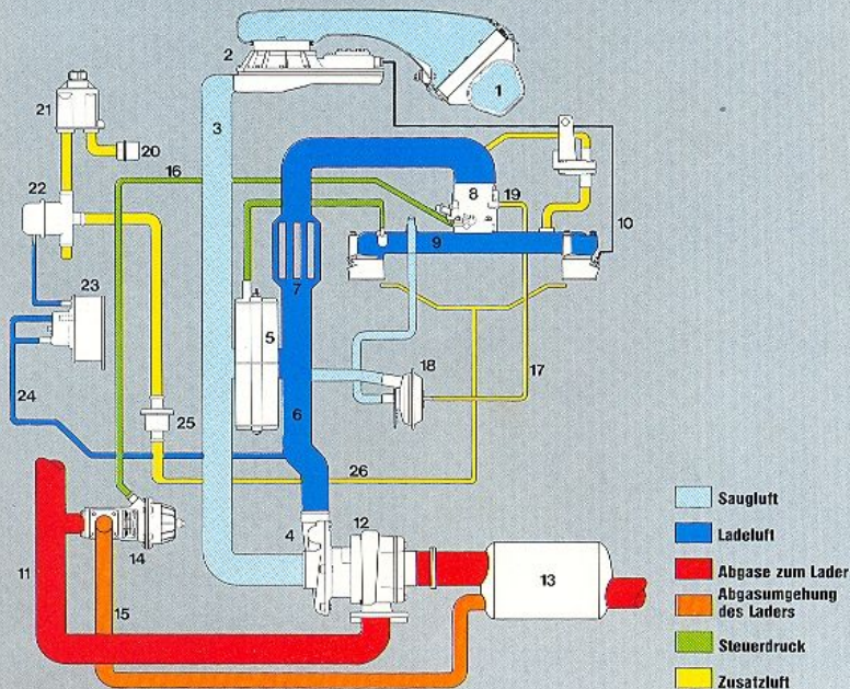
Funktionsschema
