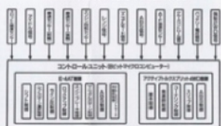
アクティブトルクスプリット4WD(E-4AT)電子制御システム
